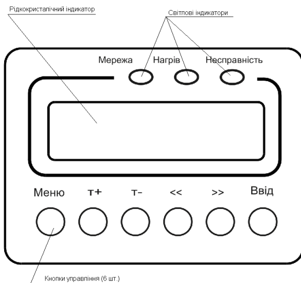
Рис. 1 Панель управління електрокотла «ТермІТ»
