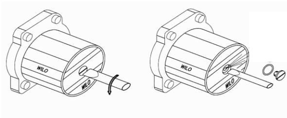
Рис. 7 Видалення повітря із циркуляційного насоса
