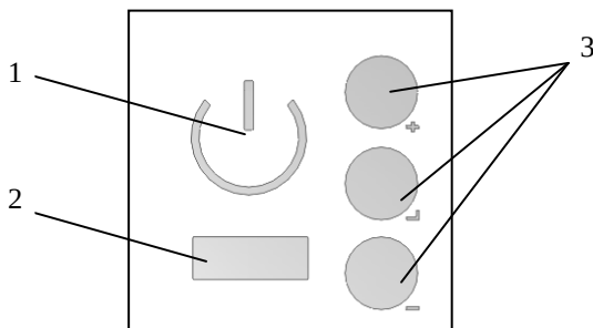
1 Вікно індикації стану електродкотла. 2 Чотирьохсимвольний LED дисплей 3 Сенсорні кнопки управління
