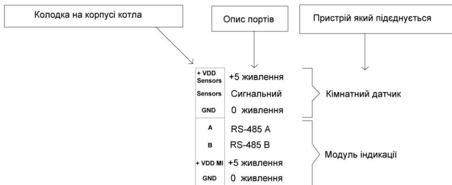
Рис. 8.1. Підключення до інтерфейсної клемної колодки.
