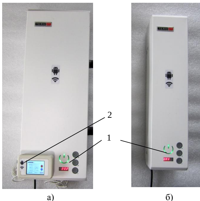
а) б) 1 Панель управління. 2 Модуль індикації та управління «ТерміТ» серії «Смарт» SMI з TFTTouchScreen дисплеєм та вбудованим датчиком кімнатної температури.
