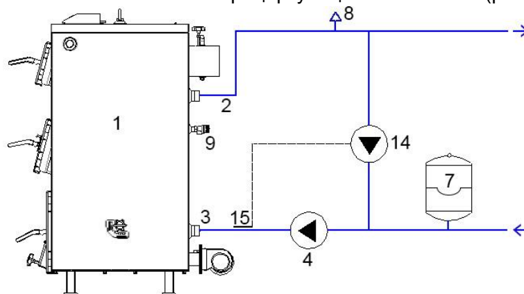
Рис.6 Схема обв'язки котла з рециркуляційним насосом (рекомендована)
