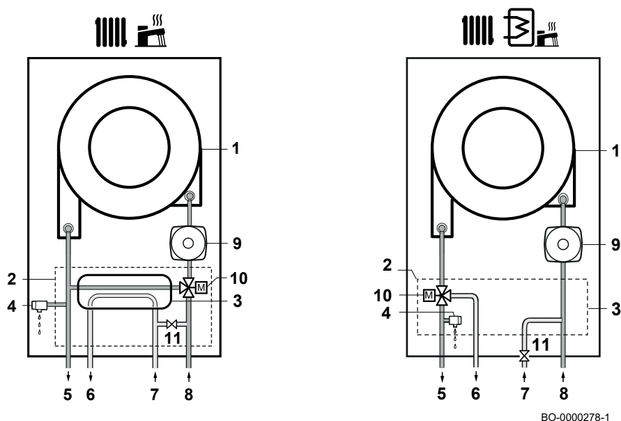
Рис. 4 Принципова схема
