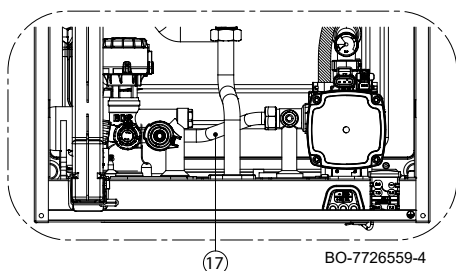
Рис. 6 Котел тільки з функцією опалення (частина, що містить блок води)
