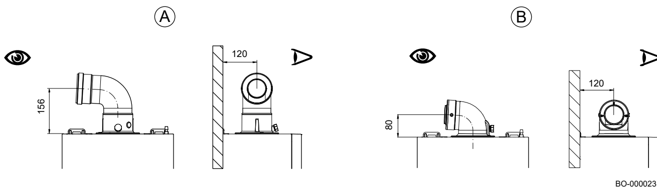
Рис. 22 Адаптер коаксіального димоходу
