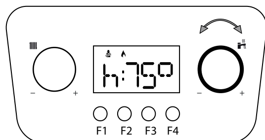
Рис. 44 Мінімальна потужність в режимі опалення
