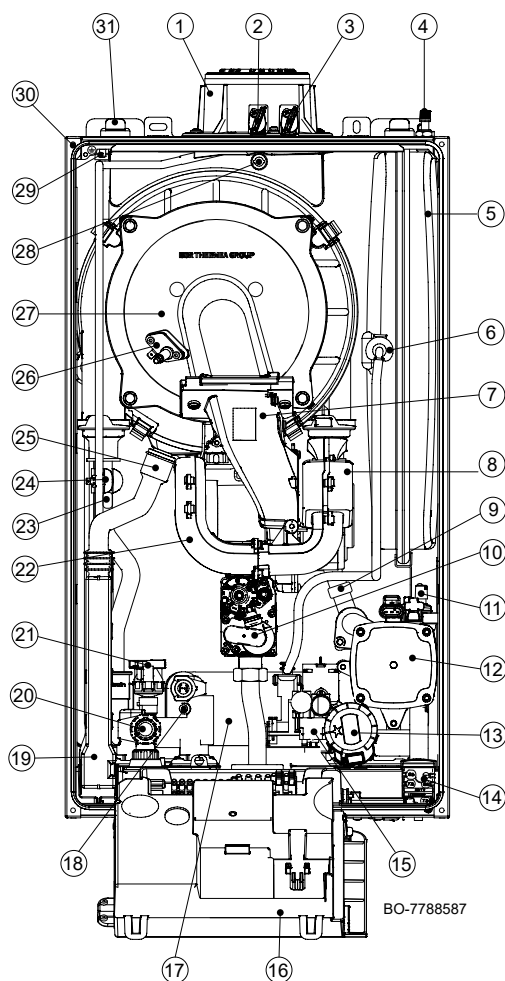
Рис. 6 Котел тільки з функцією опалення (частина, що містить блок води)
